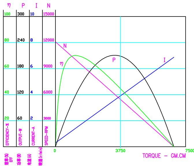
GRS-8712VFB-2376 120 V AC
